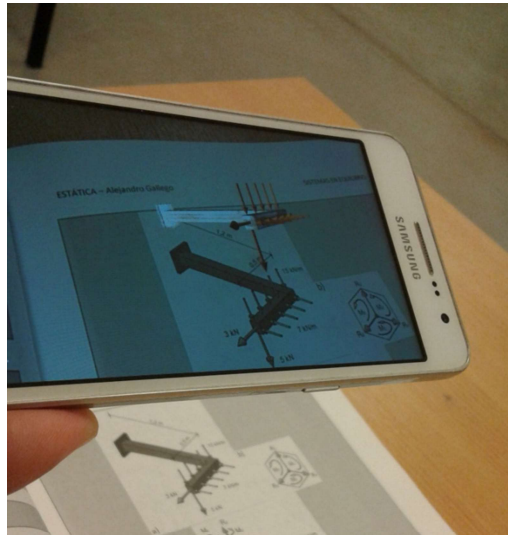
Figura 1. Ménsula con cargas [1]
