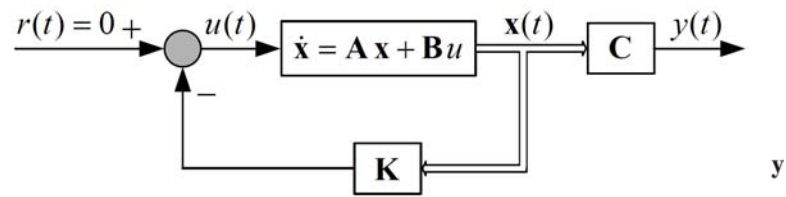
Figura 2. Sistema de control con realimentación de estados y ganancia \mathbf{K}
