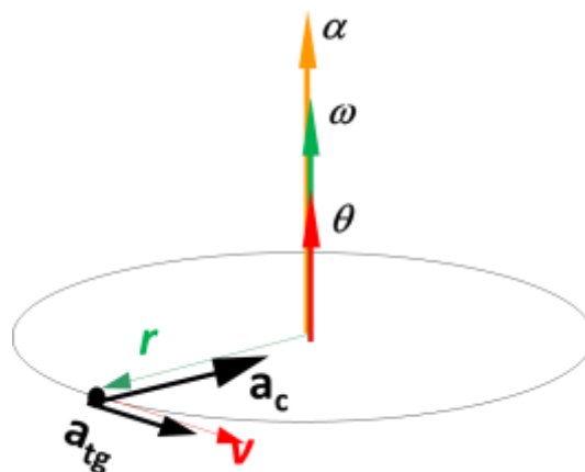
Figura 7. Relación general entre variables angulares y lineales. Fuente: elaboración propia
